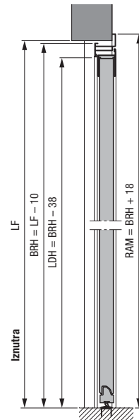
Bočna vrata s aluminijskim kutnim okvirom, profil tipa 2 Vanjski nosač
