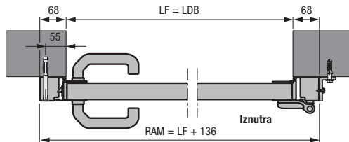
Pokrajnja vrata s aluminijskim blok okvirom, profil tipa 2 Ugradnja iza otvora
