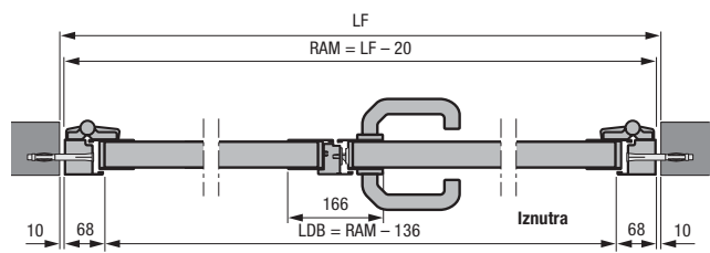
Dvokrilna bočna vrata s aluminijskim blok okvirom, profil tipa 2 Ugradnja u otvoru
