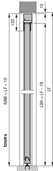
Pokrajnja vrata s aluminijskim blok okvirom, profil tipa 2 Ugradnja u otvoru
