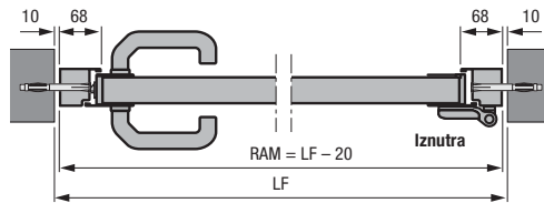
Pokrajnja vrata s aluminijskim blok okvirom, profil tipa 2 Ugradnja u otvoru
