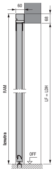
Pokrajnja vrata s aluminijskim blok okvirom, profil tipa 2 Ugradnja iza otvora
