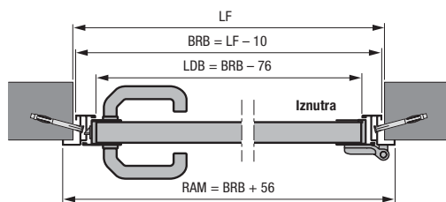
Bočna vrata s aluminijskim kutnim okvirom, profil tipa 2 Unutarnji nosač
