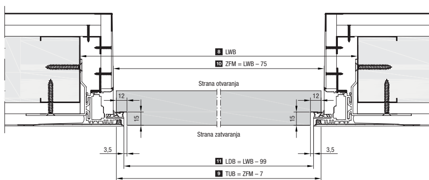
Horizontalni presjek tip RI s revers vratnim krilom
