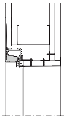
Okomiti presjek, standardno otvaranje prema van (tip NA)
