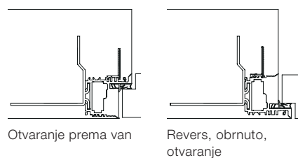
Profili Zeroline dovratnika
