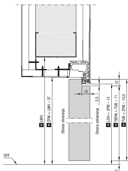
Vertikalni presjek tip RI s revers vratnim krilom
