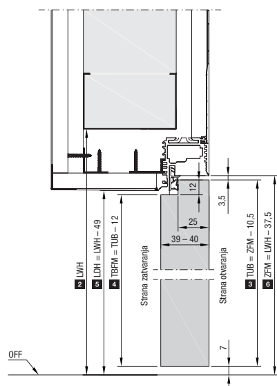
Okomiti presjek tipa NA sa vratnim krilom sa standardnim otvaranjem
