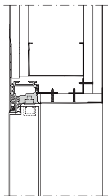
Okomiti presjek, obrnuto otvaranje u otvor vrata (tip RI)
