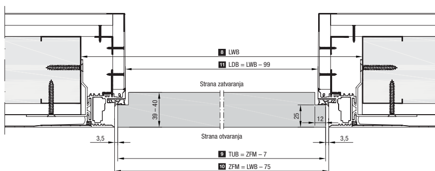
Vodoravni presjek tipa NA s vratnim krilom sa standardnim otvaranjem
